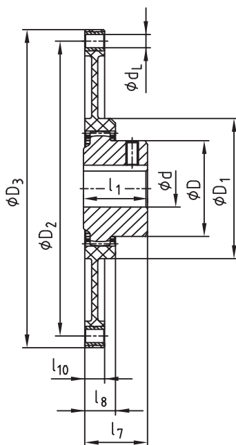
BoWex® FLE-PA dados dimensionais e técnicos
