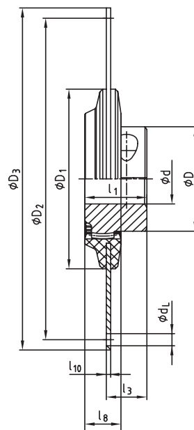
BoWex® FLE-PA dados dimensionais e técnicos
